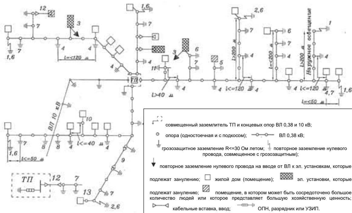
Рисунок 5.3 – Схема устройства заземления ВЛИ напряжением 0,38 кВ
