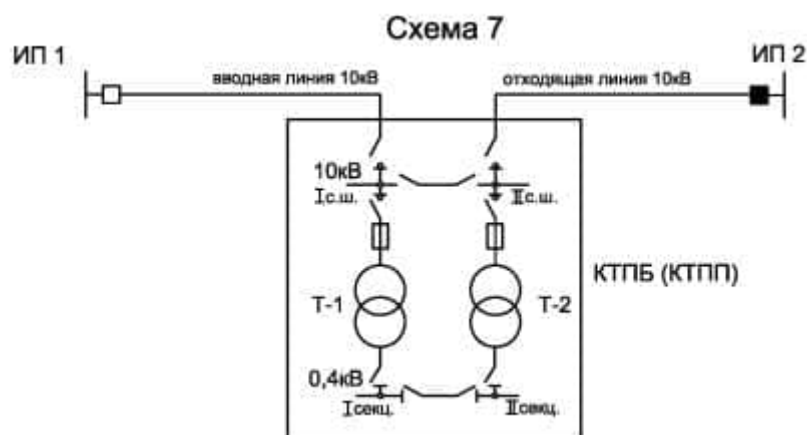
Рисунок 8.7 — Схема присоединения ТП 10/0,4 кВ, питающей потребителей категории II
