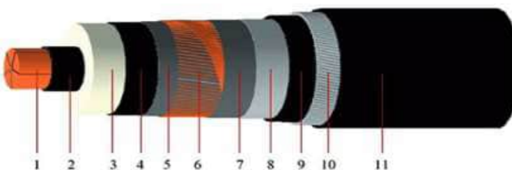
Рисунок 5.6 — Устройство одножильного кабеля из сшитого полиэтилена
