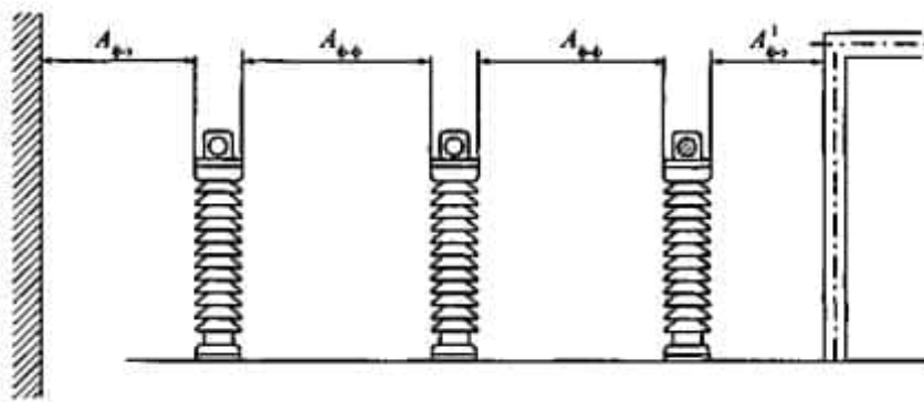
Рисунок 6.3 — Наименьшие расстояния в свету при жестких шинах между токоведущими и заземленными частями ( A_{ф-з} , A'_{ф-з} и между токоведущими частями разных фаз ( A_{ф-ф} ))
