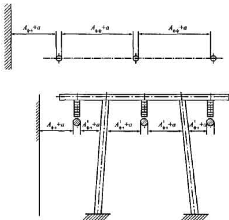
Рисунок 6.4 — Наименьшие расстояния в свету при гибких шинах между токоведущими и заземленными частями и между токоведущими частями разных фаз, расположенными в одной горизонтальной плоскости
