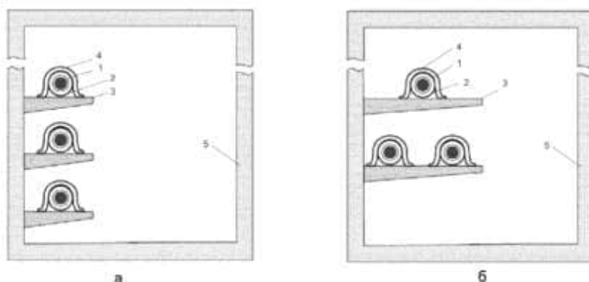
а – вертикально; б – «треугольником» с расстоянием между кабелями по воздуху. 1 – КПИ; 2 – прокладка; 3 – полка; 4 – узел крепления; 5 – туннель.
