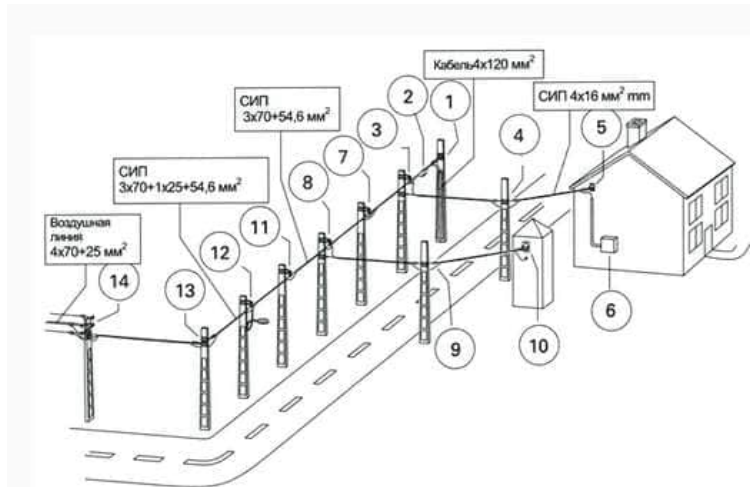
Рисунок 5.1 — Типовые узлы крепления СИП ВЛИ напряжением 0,38 кВ
