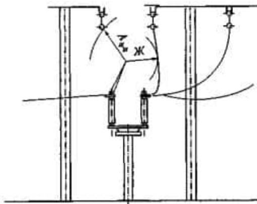
Рисунок 6.11 — Наименьшие расстояния от подвижных контактов разъединителей в отключенном положении до заземленных и токоведущих частей
