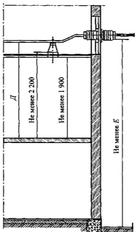
Рисунок 6.17 — Наименьшие расстояния от пола до неогражденных неизолированных токоведущих частей и до нижней кромки фарфора изолятора и высота прохода в ЗРУ. Наименьшее расстояние от земли до неогражденных линейных выводов из ЗРУ вне территории ОРУ и при отсутствии проезда транспорта под выводами
