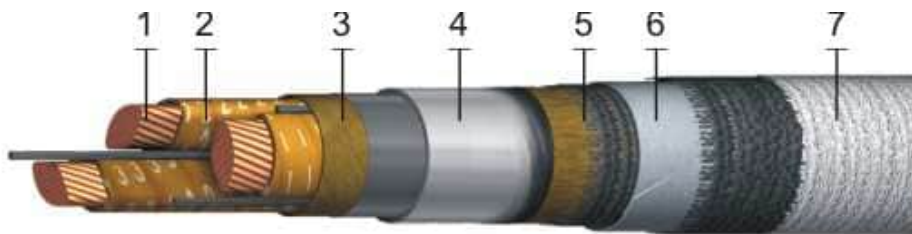
Рисунок 5.9 — Устройство кабеля с изоляцией из пропитанной бумаги
