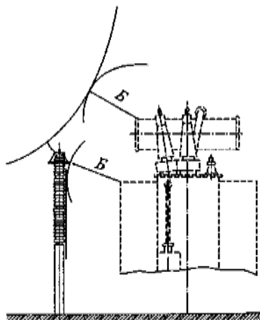
Рисунок 6.7 — Наименьшие расстояния от токоведущих частей до транспортируемого оборудования
