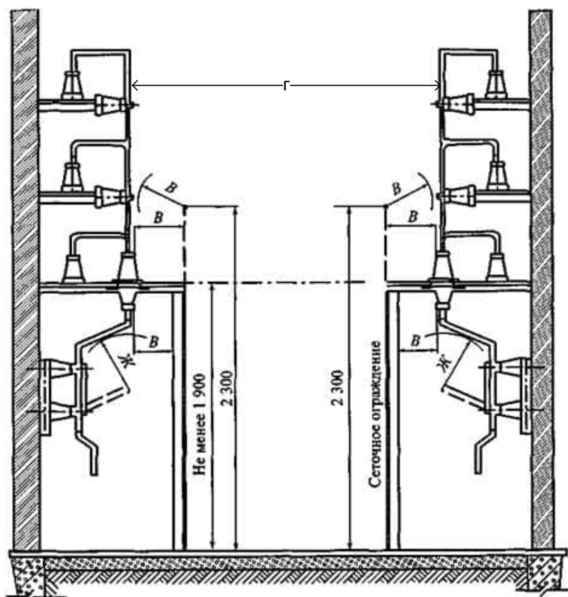
Рисунок 6.16 — Наименьшие расстояния от неизолированных токоведущих частей в ЗРУ до сетчатых ограждений и между неогражденными неизолированными токоведущими частями разных цепей (таблица 6.9)
