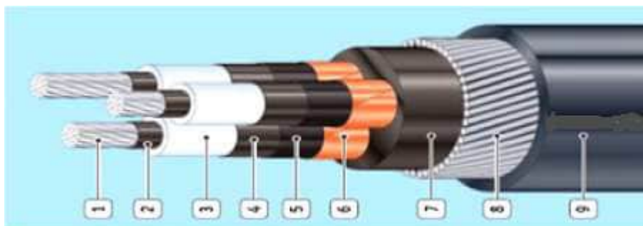
Рисунок 5.7 — Устройство одножильного кабеля из сшитого полиэтилена бронированного
