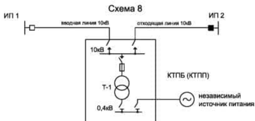
Рисунок 8.8 — Схема присоединения ТП 10/0,4 кВ, питающей потребителей категории II
