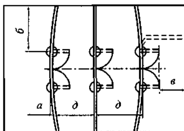
Рисунок 6.1 — Границы расположения открытых подвижных контактов разъединителя (отделителя) по отношению к заземленным и токоведущим частям
