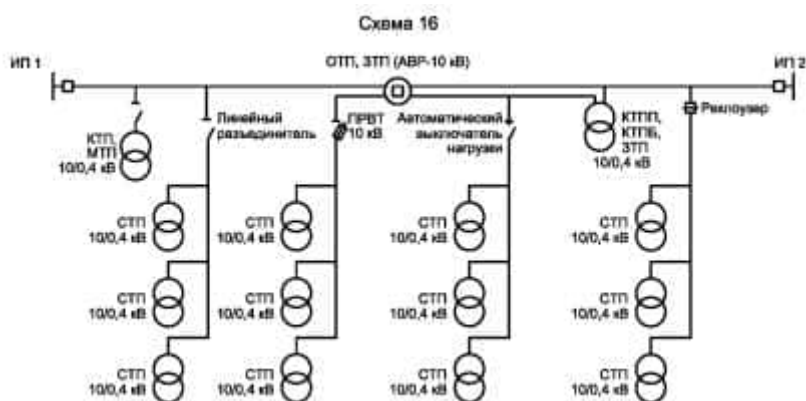
Рисунок 8.14 — Схема сети сельской РС с переносом источников трансформации (СТП 10/0,4 кВ) к потребителю в сельских населенных пунктах
