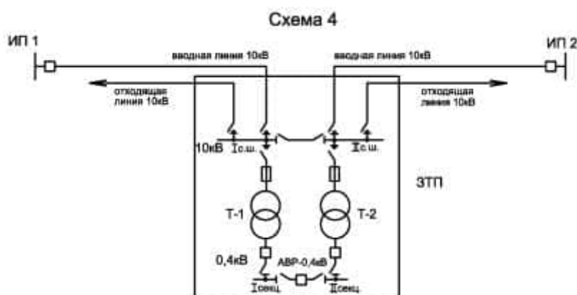
Рисунок 8.4 — Схема присоединения ТП 10/0,4 кВ, питающей потребителей категории I
