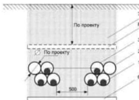
1 – КПИ; 2 – резервная ПЭ труба; 3 – ПЭ труба для фазы КПИ; 4 – бетон (по проекту); 5 – стальная труба; 6 – железобетонная плита дорожного типа (по проекту); 7 – засыпной грунт; 8 – железобетонная плита (по проекту)
