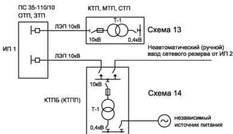
Рисунок 8.12 — Схема присоединения ТП 10/0,4 кВ, питающей потребителей категории II и III
