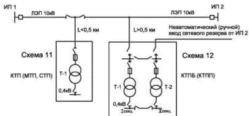
Рисунок 8.11 — Схема присоединения ТП 10/0,4 кВ, питающей потребителей категории II и III
