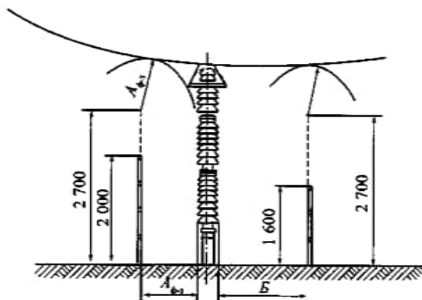
Рисунок 6.5 — Наименьшие расстояния от токоведущих частей и элементов изоляции, находящихся под напряжением, до постоянных внутренних ограждений
