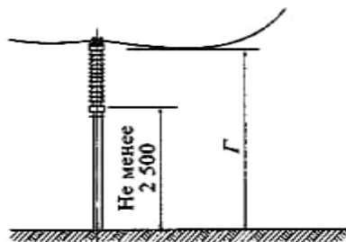
Рисунок 6.6 — Наименьшие расстояния от неогражденных токоведущих частей и от нижней кромки фарфора изоляторов до земли
