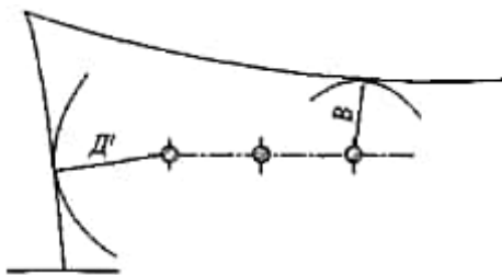
Рисунок 6.8 — Наименьшие расстояния между токоведущими частями разных цепей, расположенными в различных плоскостях с обслуживанием нижней цепи при не отключенной верхней
