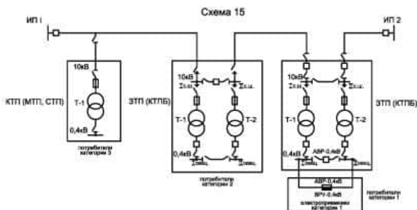
Рисунок 8.13 — Схема сети 10 кВ с подключением потребителей категории I, II и III
