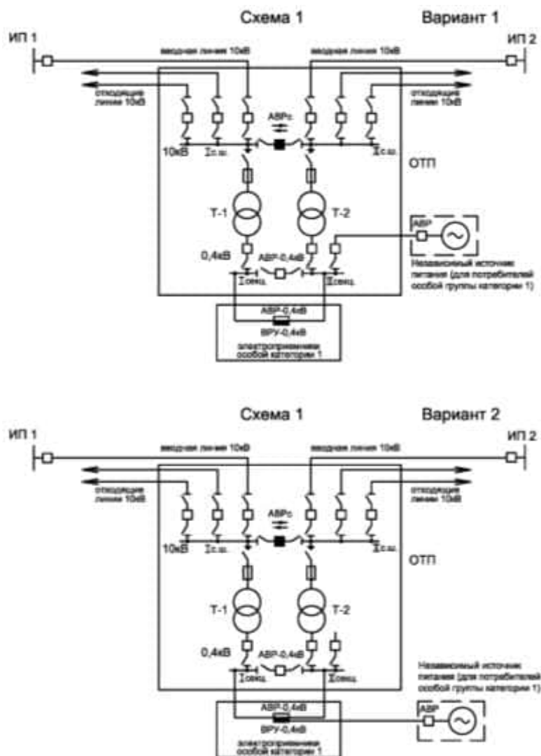
Рисунок 8.1 — Схемы вариантов присоединения ОТП 10/0,4 кВ, питающей потребителей особой группы категории I
