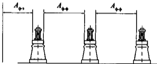
Рисунок 6.14 — Наименьшие расстояния в свету между неизолированными токоведущими частями разных фаз в ЗРУ и между ними и заземленными частями (таблица 6.9)
