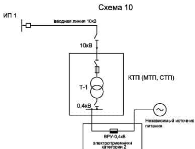
Рисунок 8.10 — Схема присоединения ТП 10/0,4 кВ, питающей потребителей категории II
