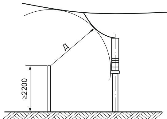
Рисунок 6.10 — Наименьшие расстояния от токоведущих частей до верхней кромки внешнего ограждения
