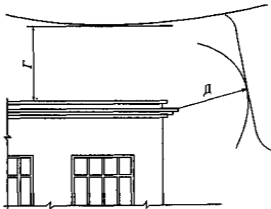
Рисунок 6.12 — Наименьшие расстояния между токоведущими частями и зданиями и сооружениями
