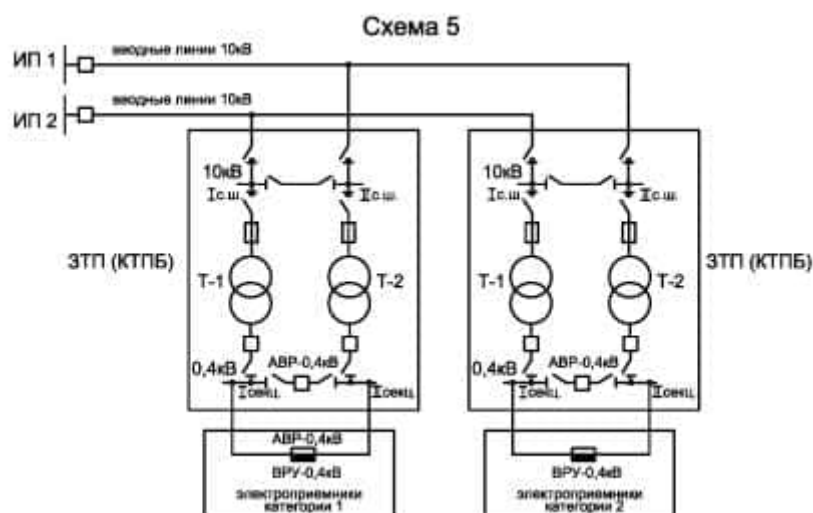
Рисунок 8.5 — Схема присоединения ТП 10/0,4 кВ, питающей потребителей категории I и II
