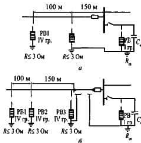
Рисунок 6.21 — Схемы защиты электродвигателей мощностью до 3 МВт при подходе ВЛ на деревянных опорах
