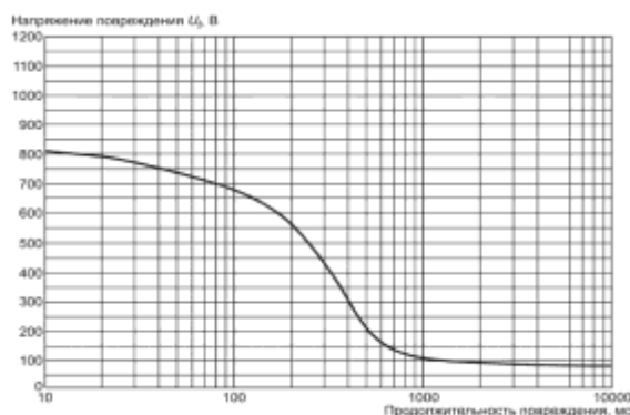
Рисунок Б.2 — Допустимое напряжение повреждения в системе низкого напряжения при замыкании на землю в системе высокого напряжения
