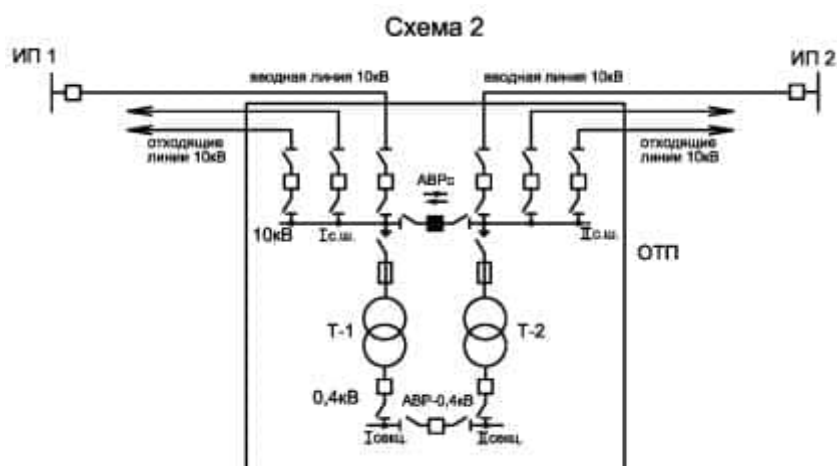
Рисунок 8.2 — Схема присоединения ТП 10/0,4 кВ, питающей потребителей категории I
