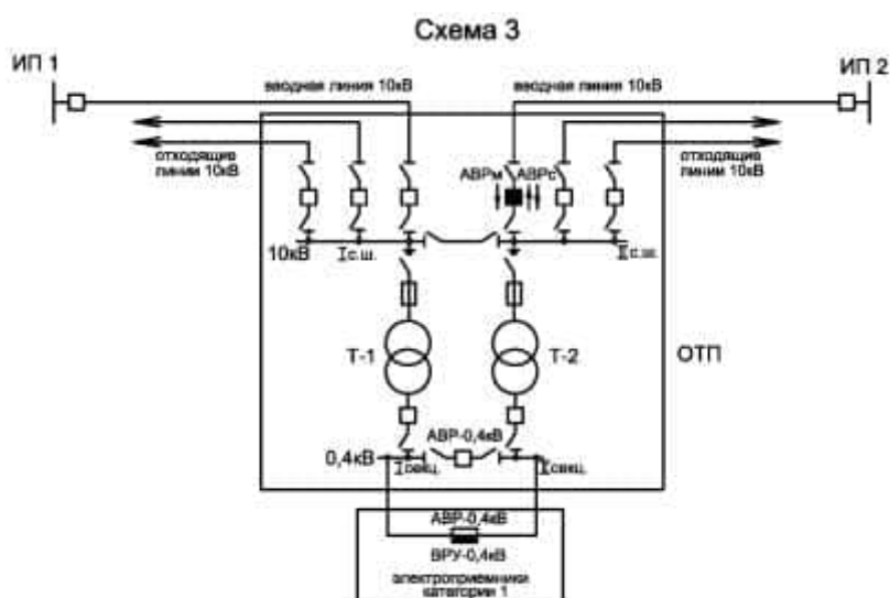
Рисунок 8.3 — Схема присоединения ТП 10/0,4 кВ, питающей потребителей категории I
