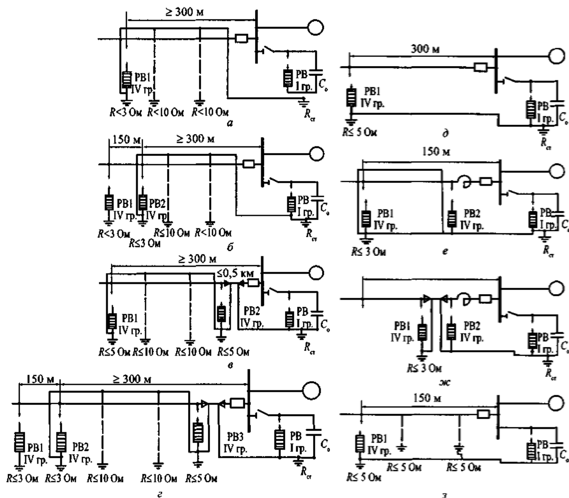
Рисунок 6.20 — Схемы защиты вращающихся электрических машин от грозовых перенапряжений
