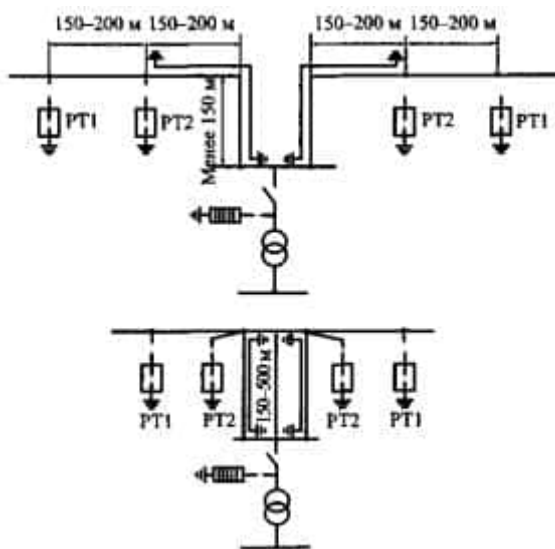
Рисунок 6.19 — Схемы защиты от грозовых перенапряжений ПС, присоединенных к ВЛ с помощью заходов длиной до 150 и более 150 м
