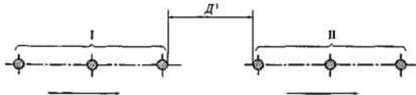
Рисунок 6.9 — Наименьшие расстояния по горизонтали между токоведущими частями разных цепей с обслуживанием одной цепи при неотключенной другой
