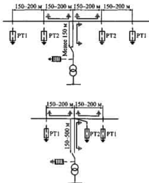
Рисунок 6.18 — Схемы защиты от грозовых перенапряжений ПС, присоединенных к ВЛ ответвлениями длиной до 150 и более 150 м
