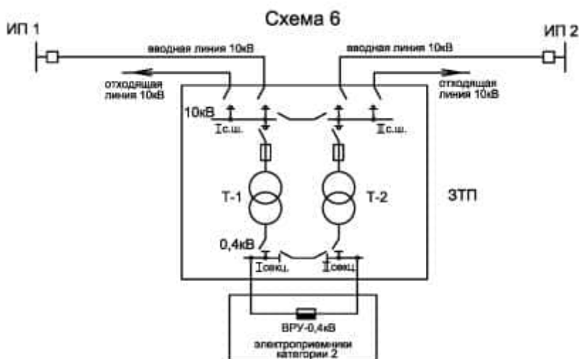
Рисунок 8.6 — Схема присоединения ТП 10/0,4 кВ, питающей потребителей категории II
