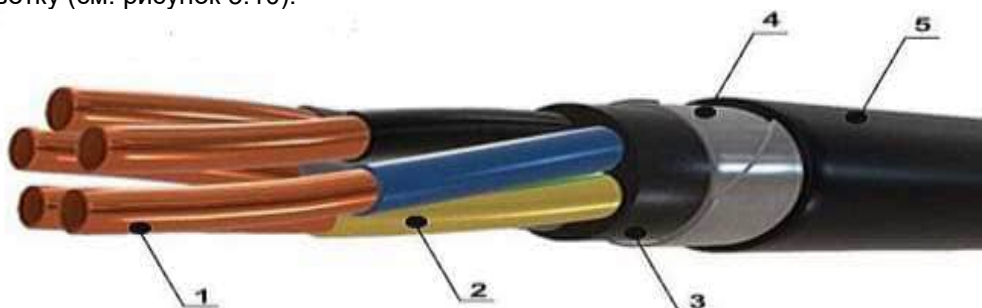
1 – медная токопроводящая жила; 2 – изоляция из ПВХ пластиката; 3- оболочка из ПВХ пластиката; 4 – броня из стальных лент; 5 – выпрессованный защитный шланг из ПВХ
