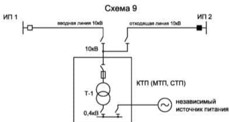
Рисунок 8.9 - Схема присоединения ТП 10/0,4 кВ, питающей потребителей категории II
